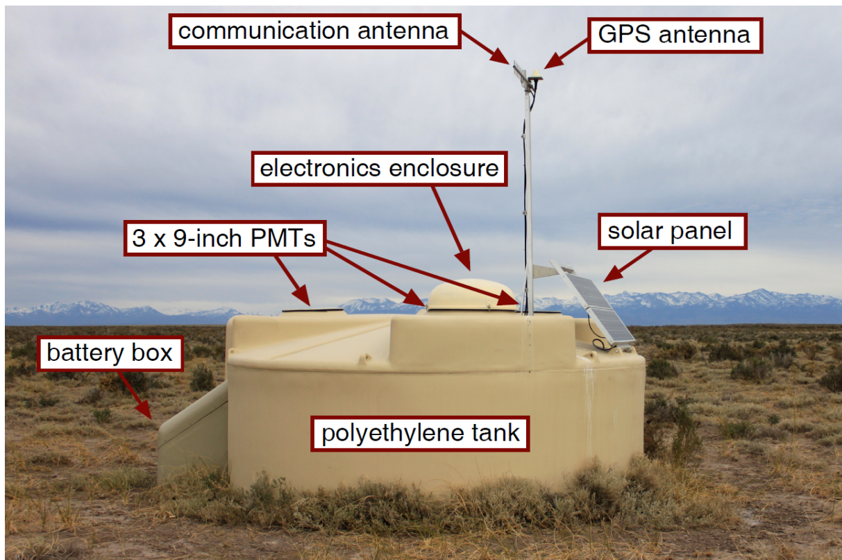
Figura 2.1.1: Detectores Cherenkov en Agua en el Observatorio Pierre Auger junto a sus componentes principales. Obtenido de [14]
