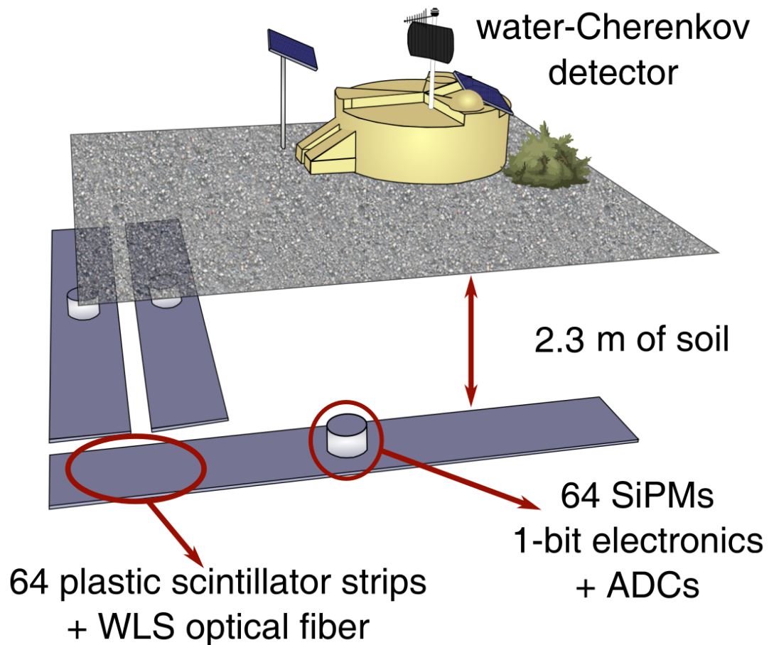
Figura 2.4.1: Esquema de Detector Subterráneo de Muones junto a su estación de superficie asociada donde se observa la distribución de los tres módulos centelladores. Obtenido de [14].
