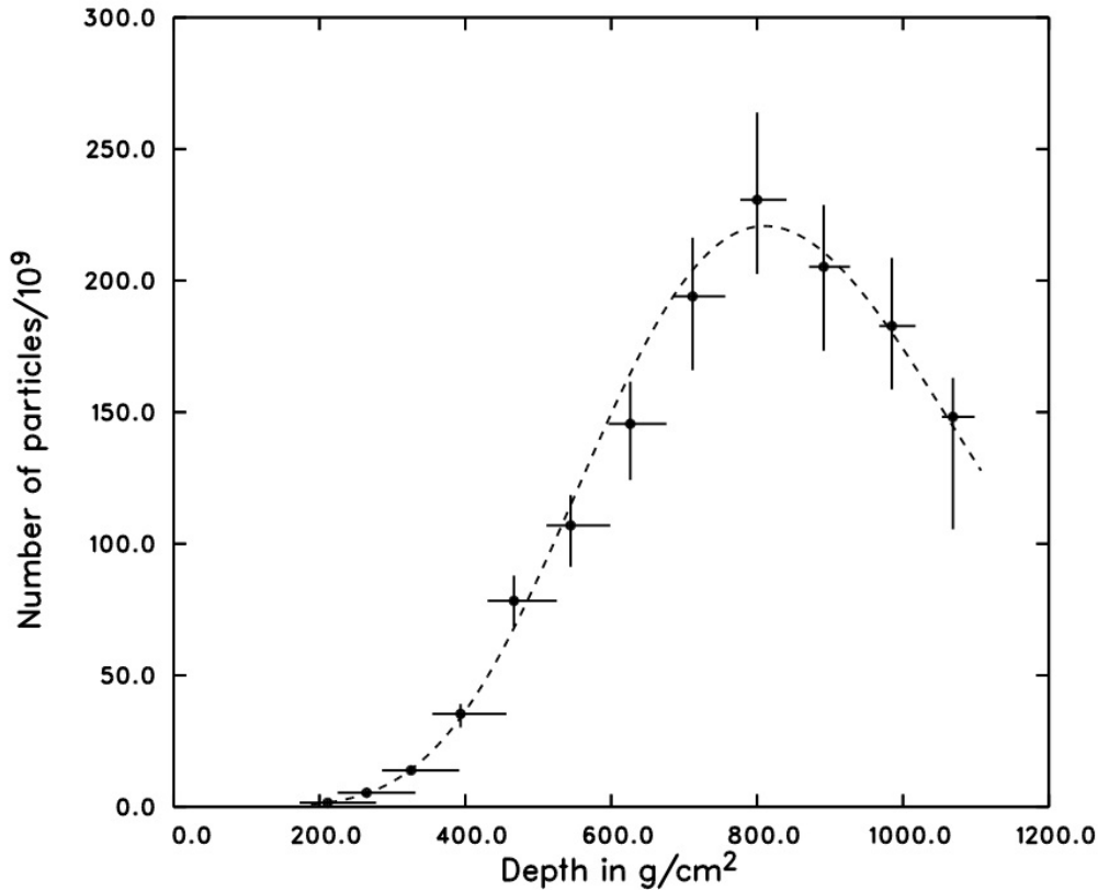
Figura 5.6.2: El gráfico corresponde al evento de mayor energía detectado por el experimento Fly's Eye ( E \approx 3,2 \times 10^{20} eV) extraído de [38]. Se observa claramente la fase de multiplicación hasta alcanzar la profundidad del máximo, seguida de la atenuación de la cascada. La distancia recorrida de atmósfera hasta llegar al máximo es lo que se denomina X_{max} .
