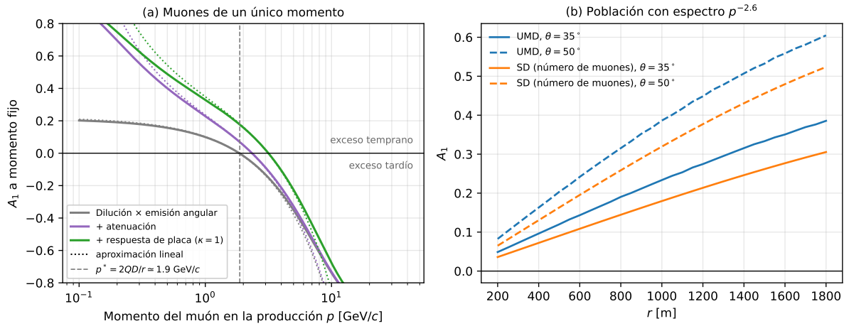
Figura 3.4.1: Modelo de juguete de la Ec. 3.4.1 ( D = 7,5 km, Q = 0,15 GeV/c, \gamma = 2,6 ). (a) Asimetría de muones de un único momento de producción en el punto de referencia ( r = 1200 m, \theta_{sh} = 35^\circ ): sólo dilución y emisión angular (gris), con atenuación (violeta) y con la respuesta de un detector plano ( \kappa = 1 ). Las líneas punteadas son la aproximación lineal de la Ec. 3.4.6, y la línea a trazos marca el momento de cruce p^* = 2QD/r . (b) Asimetría de una población en función del radio, para el conteo del UMD (azul) y el número de muones que entran en un tanque del SD (naranja), para \theta_{sh} = 35^\circ (líneas llenas) y 50^\circ (a trazos).
